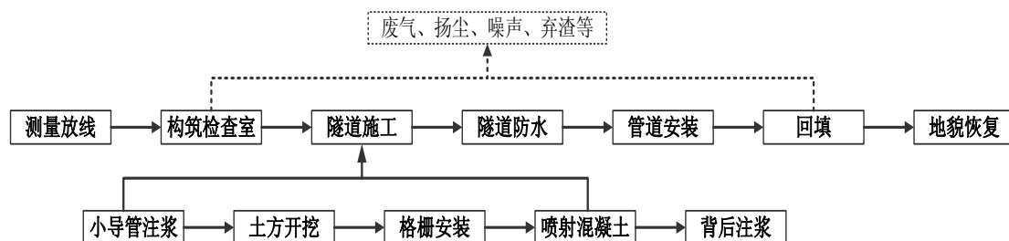
图 3 管线施工工艺流程
