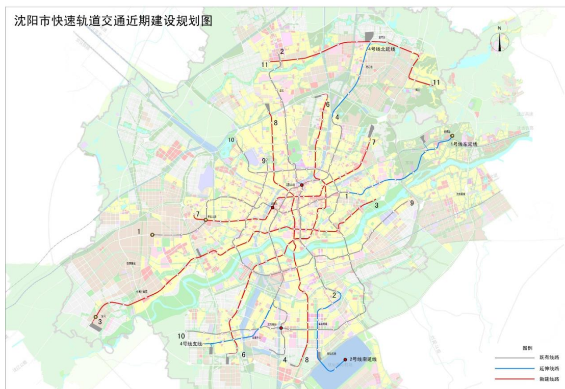
图2 近期建设规划车辆段及停车场示意图
