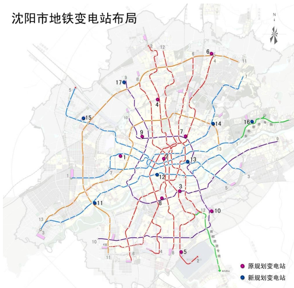
图3 沈阳市地铁变电站布局
