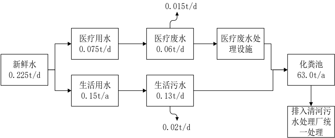
图 5-2 本项目水平衡图
