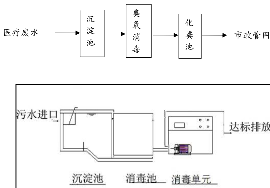
图7-1 污水处理设备工艺流程及结构图
