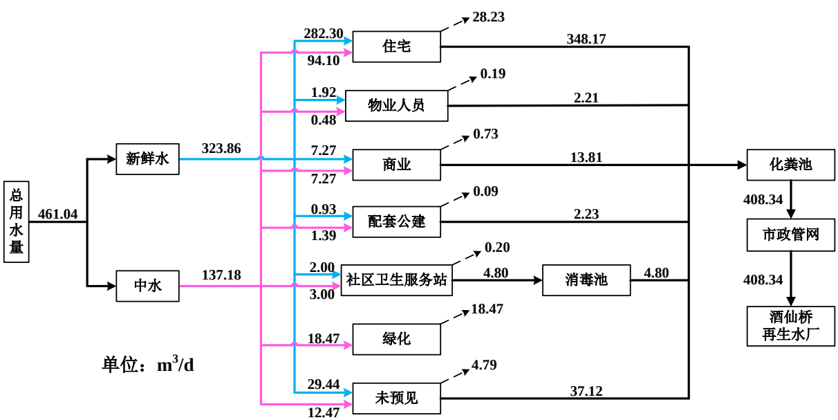
图 4 项目水平衡图
