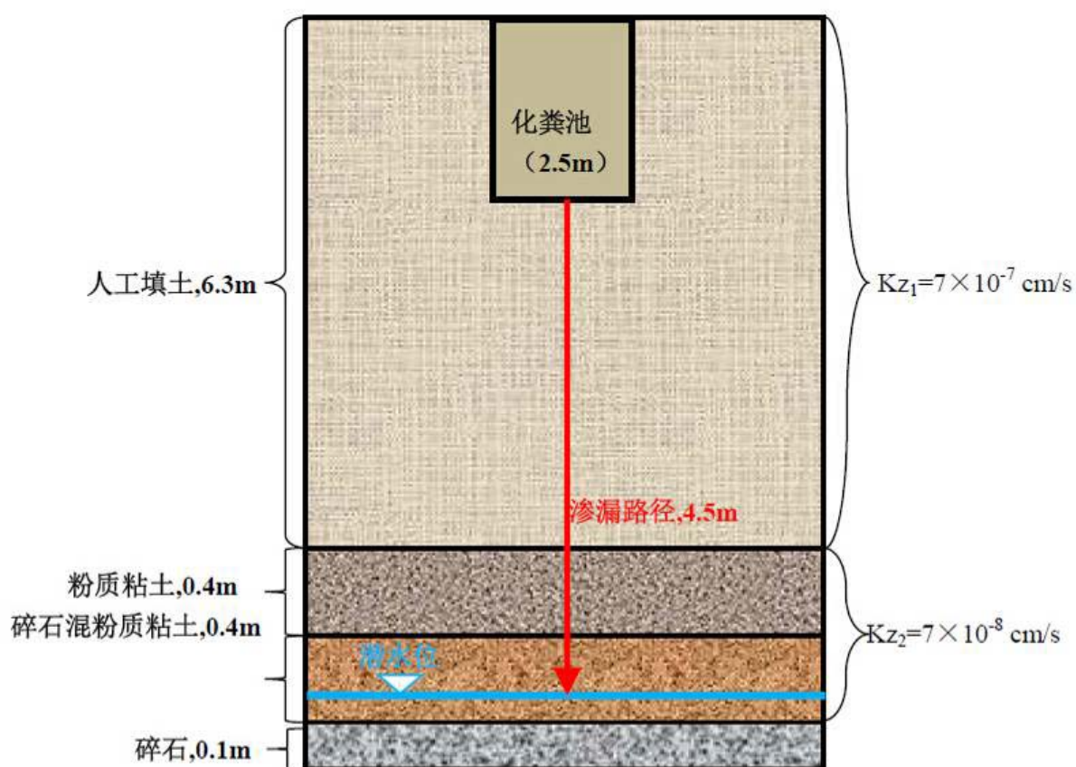
图 5 项目区附近地层概况
