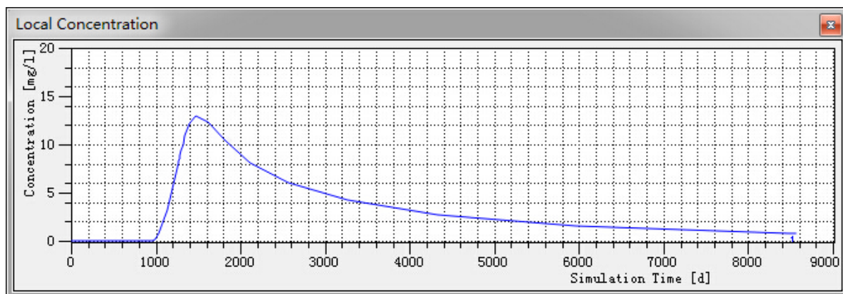
图 4.3-10 基坑南侧观测井 COD 浓度变化曲线
