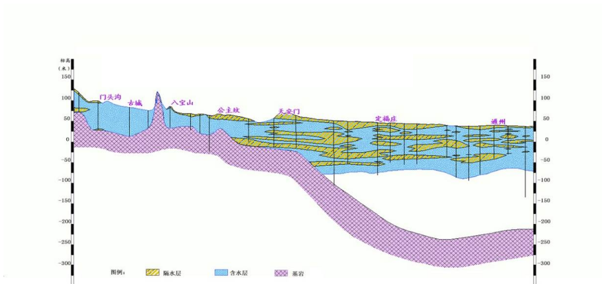
图 4.3-3 通州至门头沟水文地质剖面图
