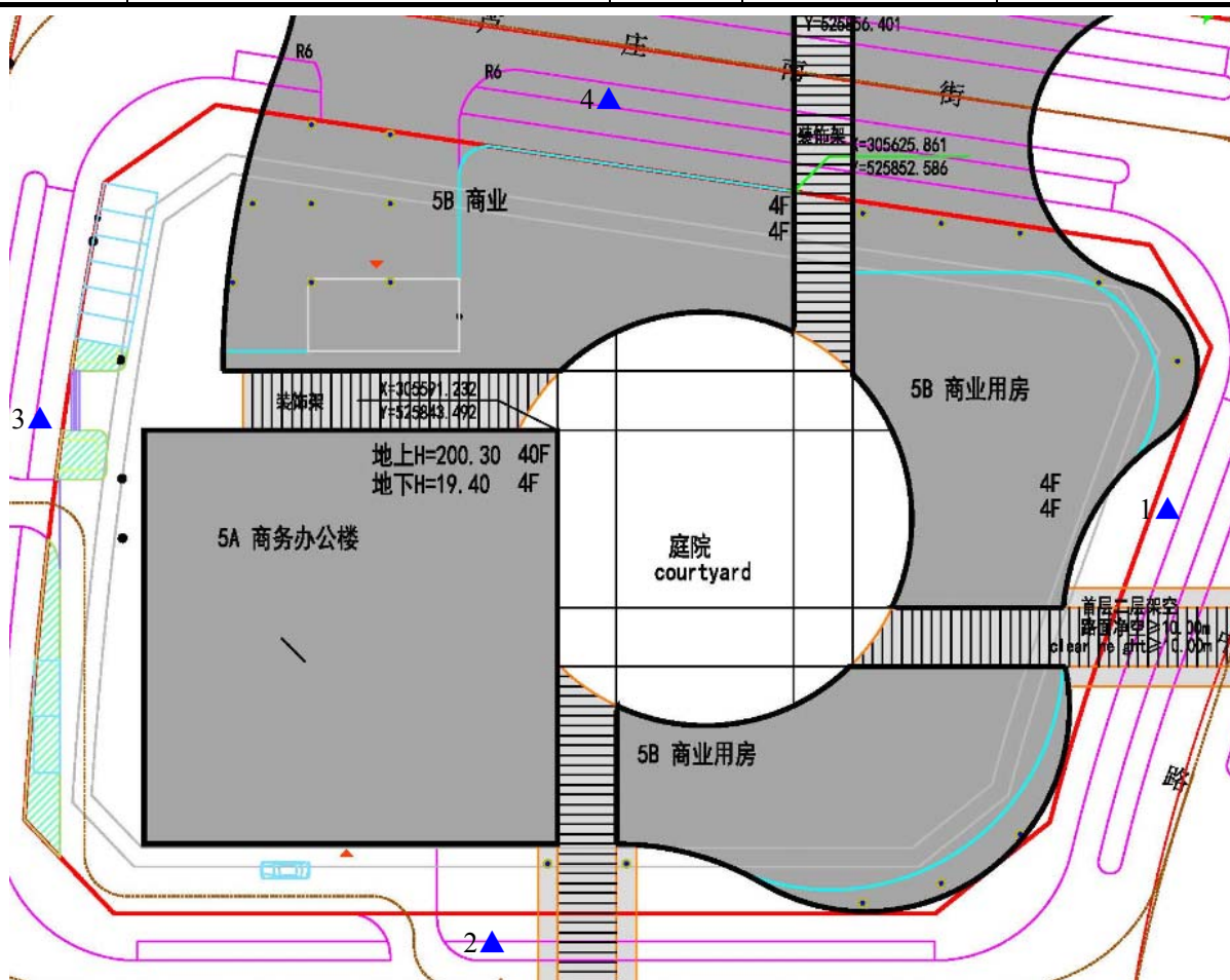
图 3.4-3 噪声监测点位示意图
