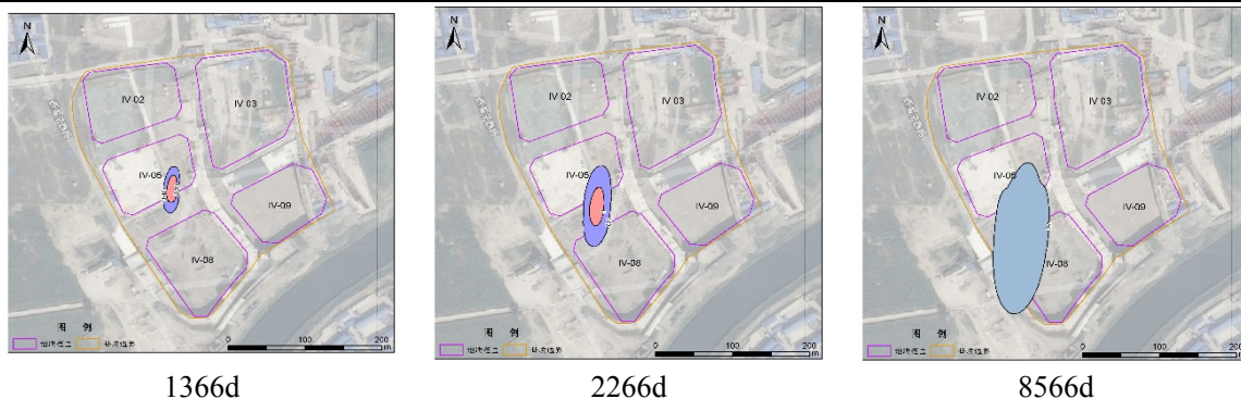
图 4.3-9 化粪池发生渗漏，不同时期 COD 运移浓度范围
