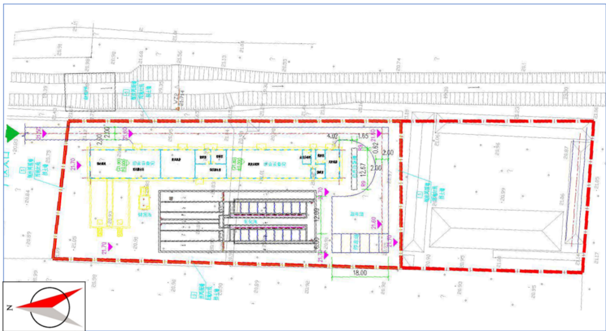
2.1-1 厂区总平面布置图
