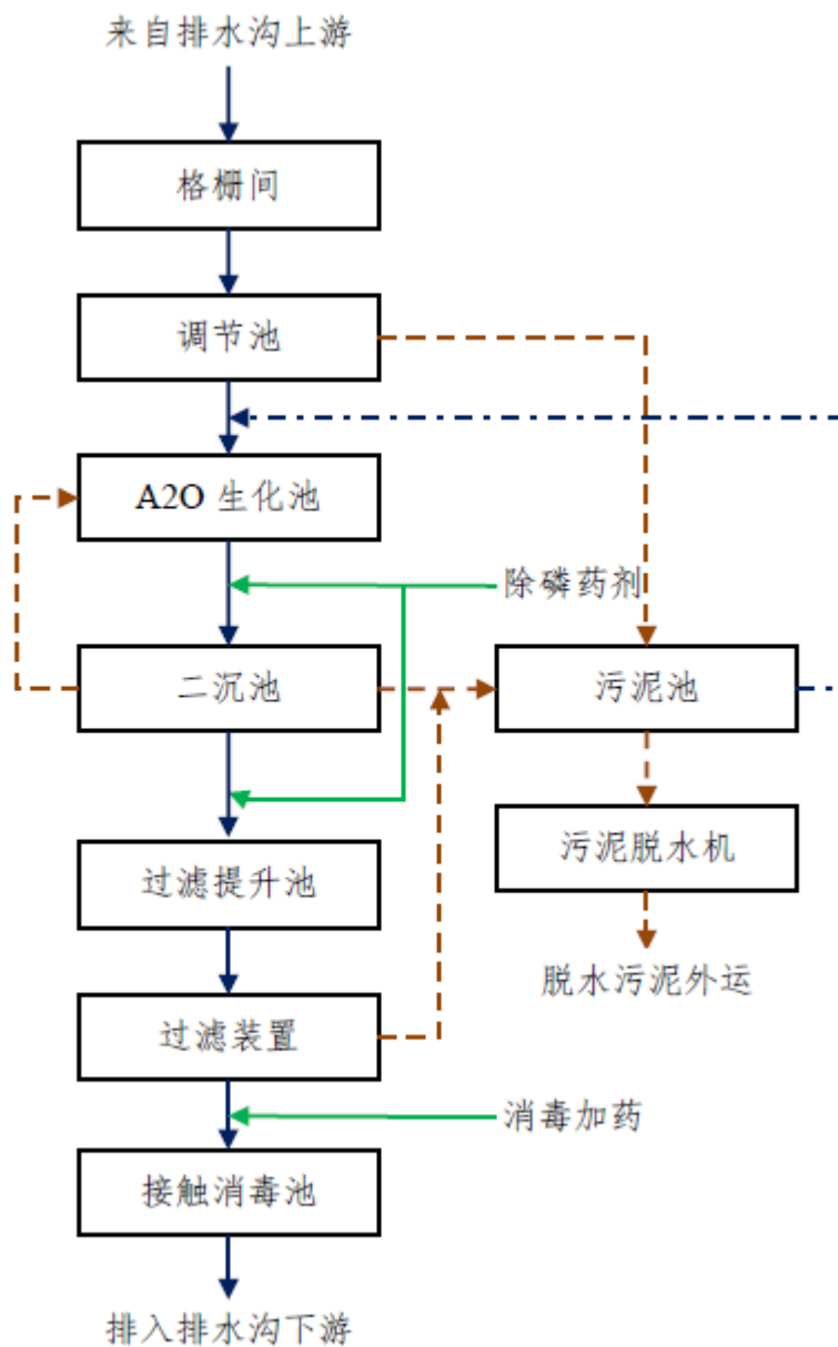
图 2.3-1 三支边沟污水处理站工艺流程图
